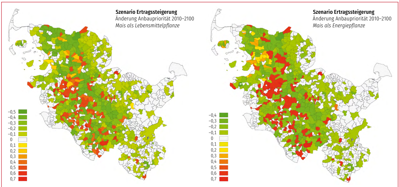
Abb.2: Veränderungen der Flächenprioritäten (prozentuale Änderungen/100) für den Anbau von Mais für Nahrung (links) oder Energie (rechts) in den Gemeinden Schleswig-Holsteins zwischen 2010 und 2100 (Yang 2016). Quelle: Eigene Darstellung
